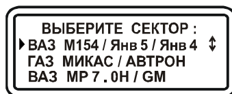
Рис. 5 Выбор микропрограммы
